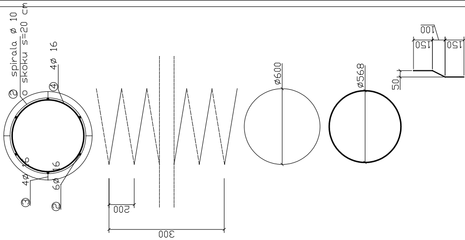
PRZĘKRÓJ POPRZECZNY PALA
