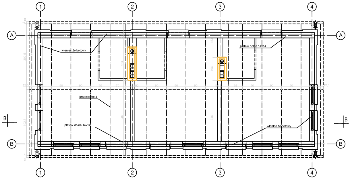
RZUT WIĘŻBY
