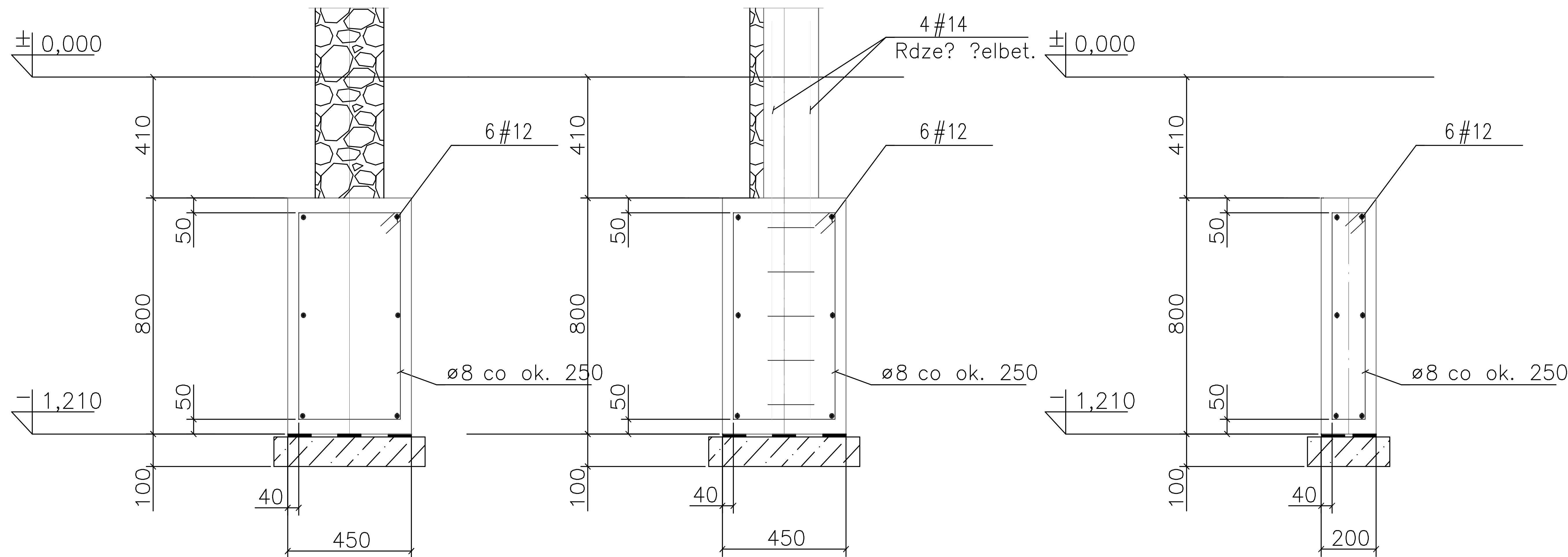
PRZEKR?J 1 - 1 PRZEKR?J 2 - 2
