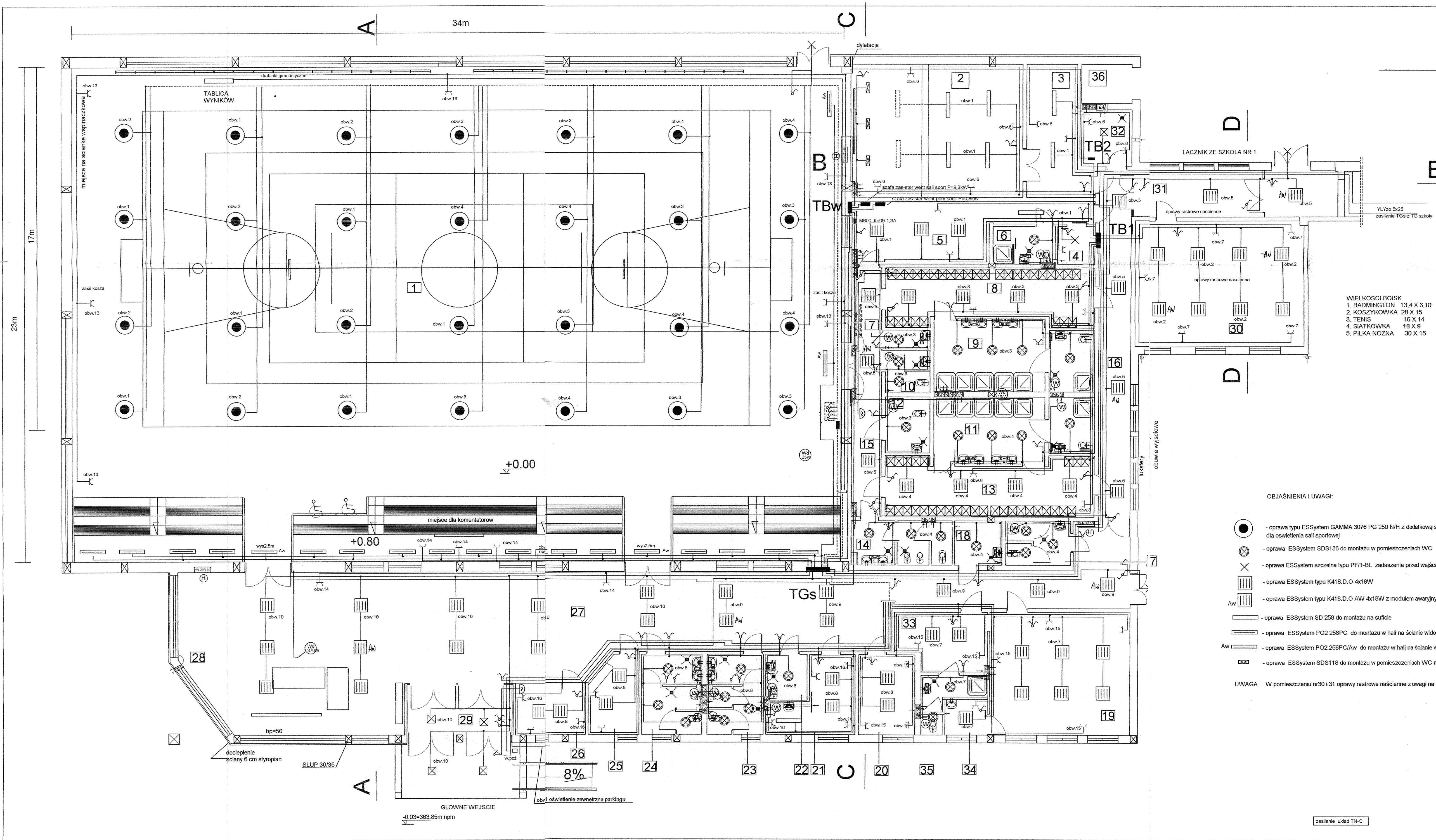
RZUT PRZYZIEMIA SKALA 1:100
