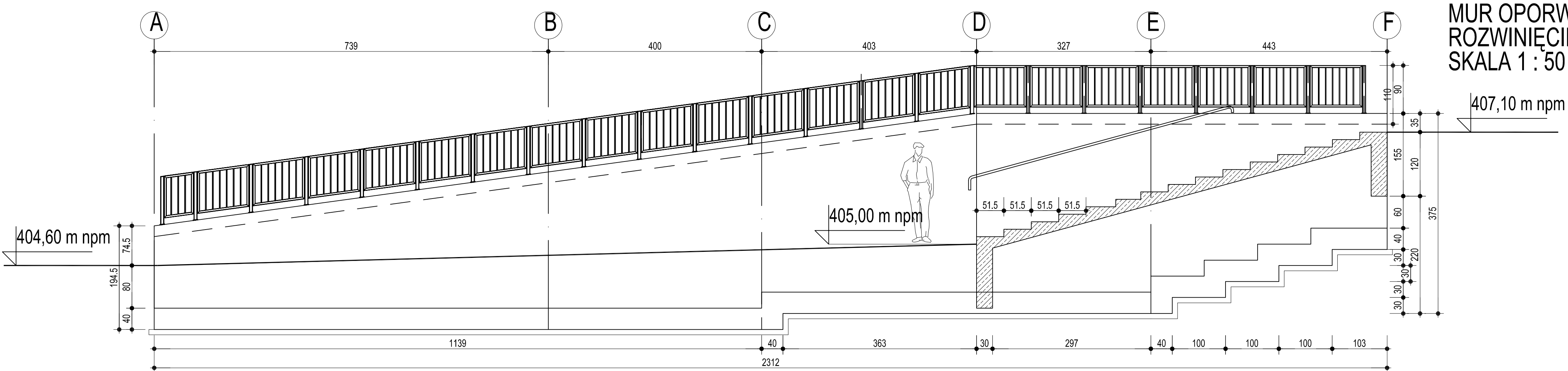
MUR OPORWY ROZWINIĘCIĘ W OSI A1 - F1 SKALA 1 : 50
