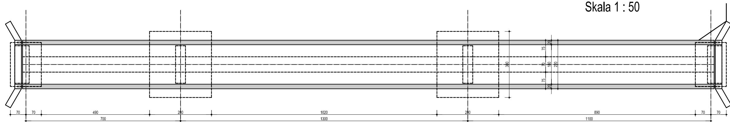
KŁADKA DLA PIESZYCH RZUT Z GÓRY Skala 1 : 50
