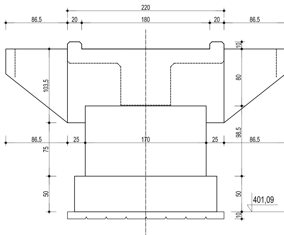
KŁADKA DLA PIESZYCH PODPORA SKRAJNA - SZT. 2 Skala 1 : 25
