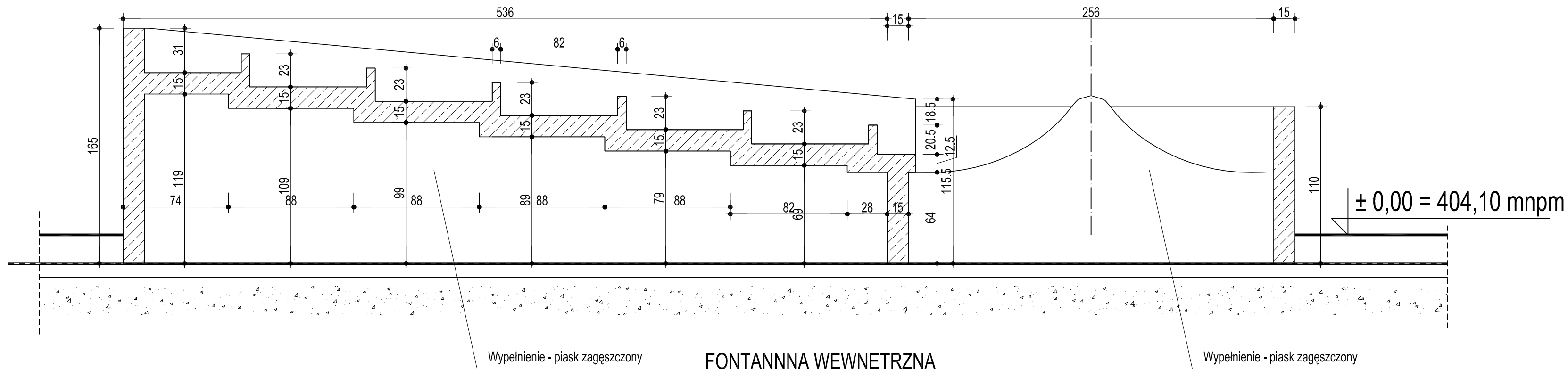
FONTANNNA WEWNĘTRZNA PRZEKRÓJ PODŁUŻNY Skala 1 : 50
