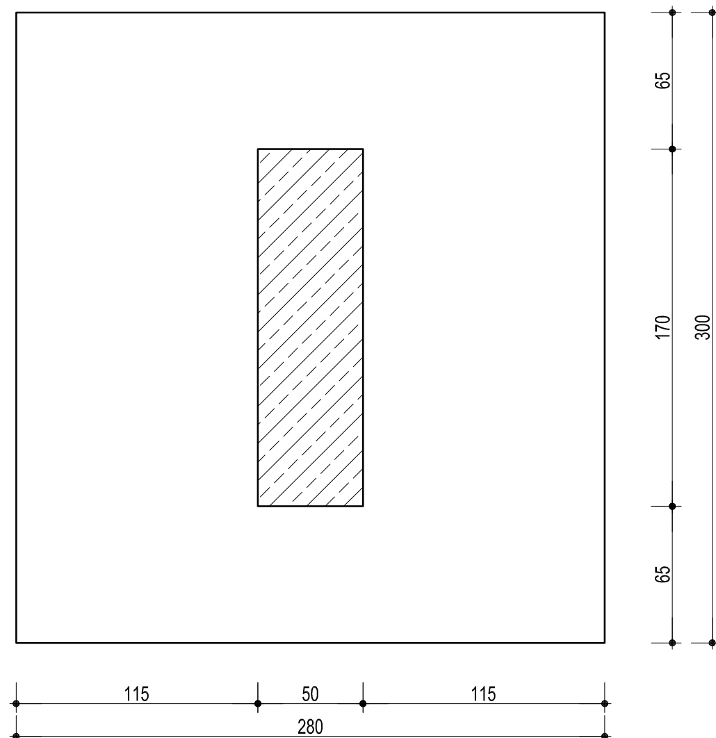
KŁADKA DLA PIESZYCH PODPORA ŚRODKOWA - SZT. 2 Skala 1 : 25
