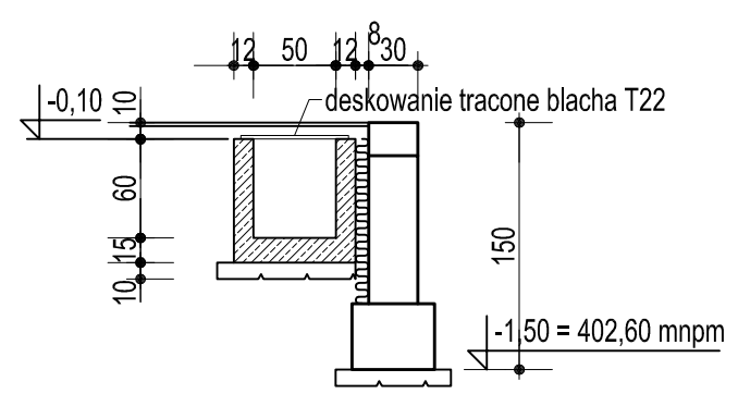
PRZĘKRÓJ a - a 1 : 50
