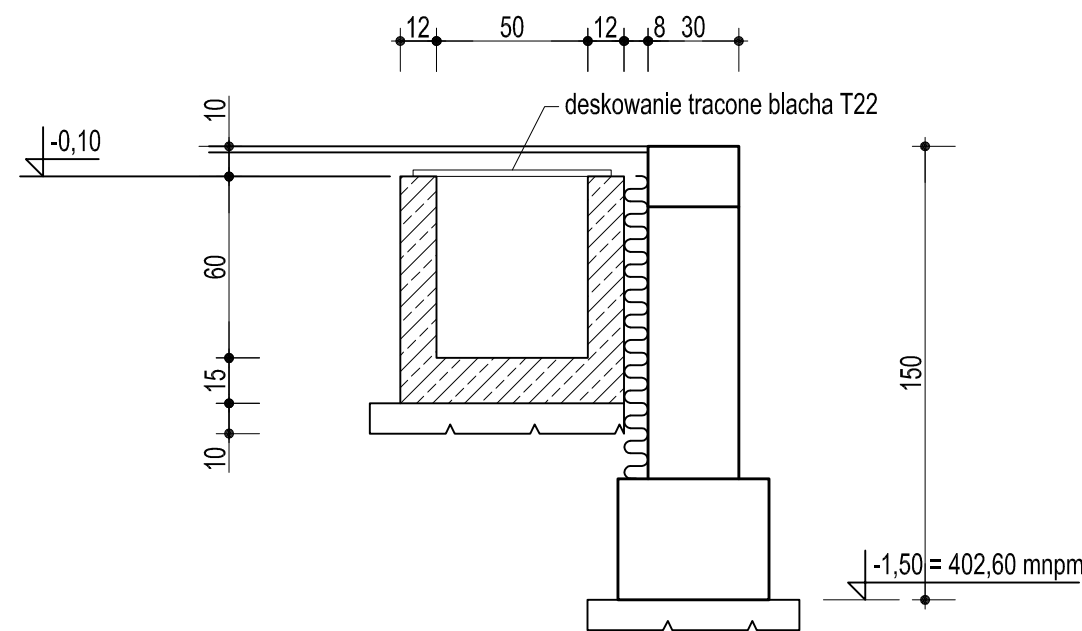
PRZĘKRÓJ a - a 1 : 25
