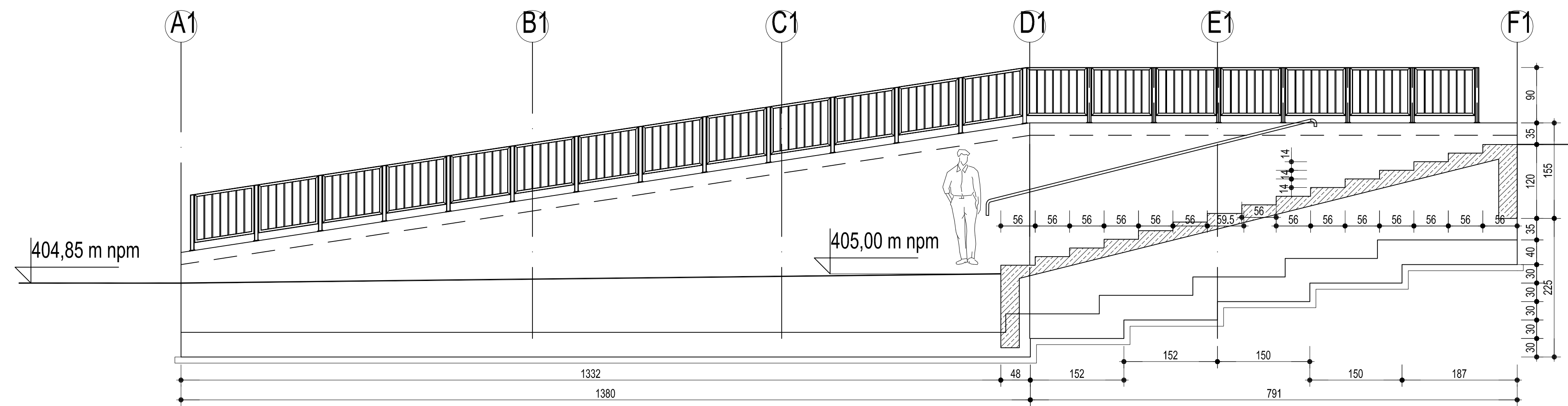
MUR OPORWY ROZWINIĘCIĘ W OSI A1 - F1 SKALA 1 : 50
