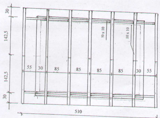
Rzut więźby
