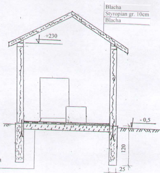
Przekrój A-A
