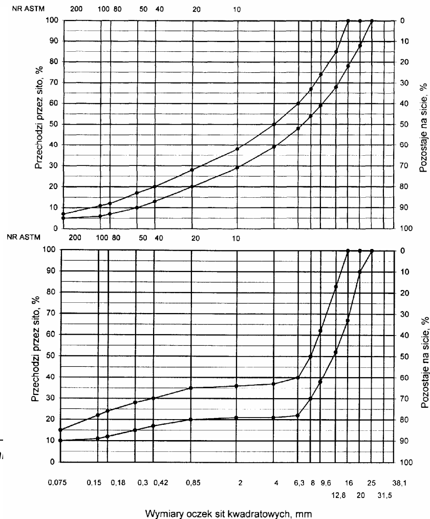
Rys. 4. Krzywe graniczne uziarnienia mieszanki mineralnej BA od 0 do 20 mm do warstwy ścieralnej nawierzchni drogi o obciążeniu ruchem od KR3 do KR6
