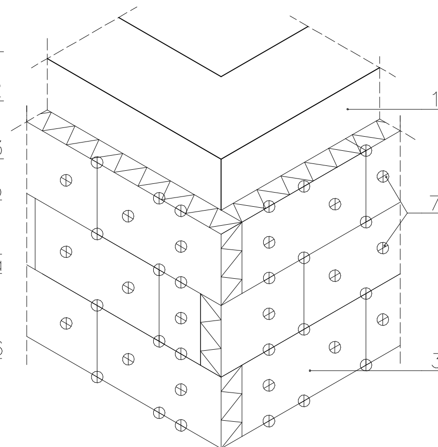
3. UKŁAD PŁYT STYROPIANOWYCH I KOŁKÓW
