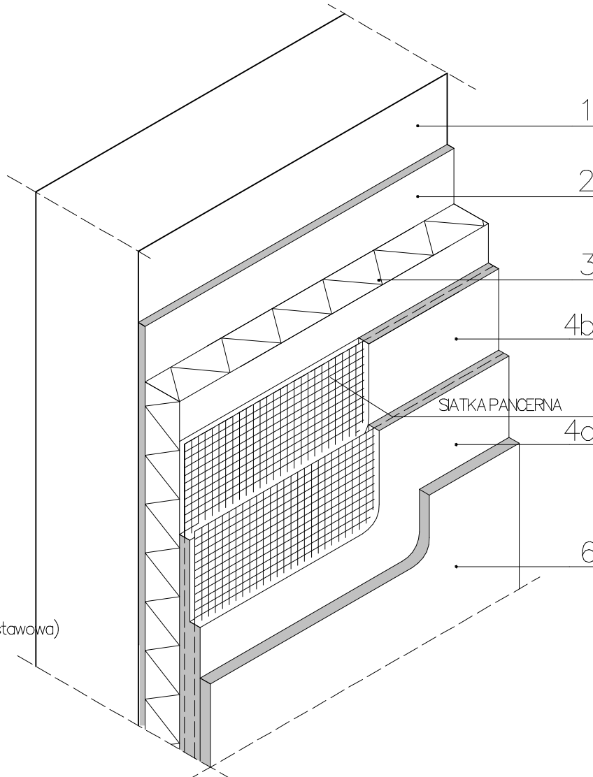
2. "B" – UKŁAD WARSTW OCEPLAJĄCYCH – WZMOCNIONY –
