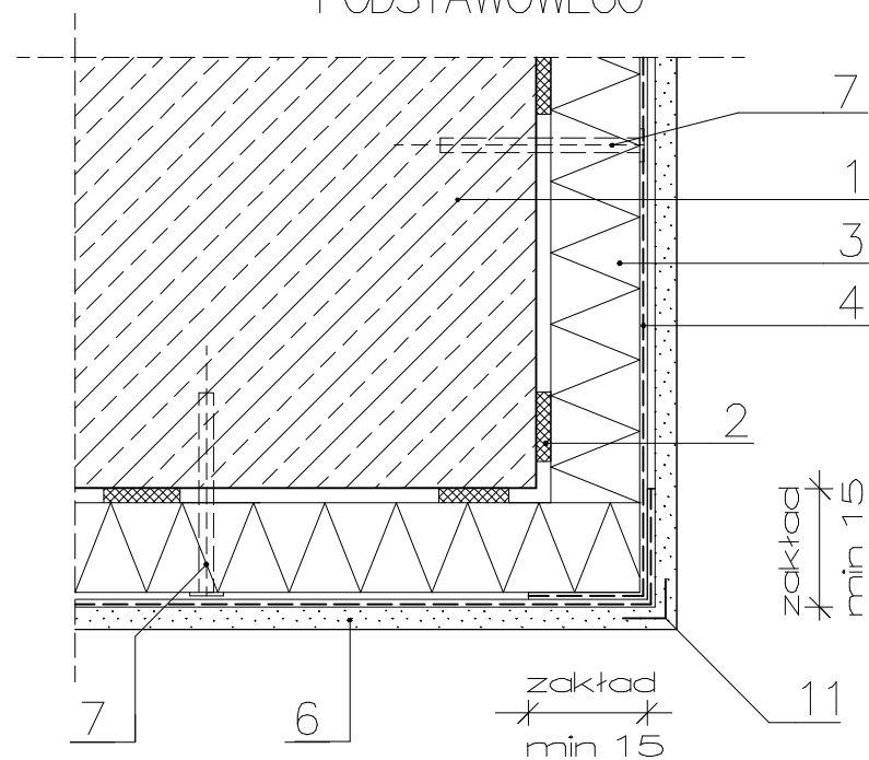
4. NAROŻE NA WYSOKOŚCI UKŁADU PODSTAWOWEGO
