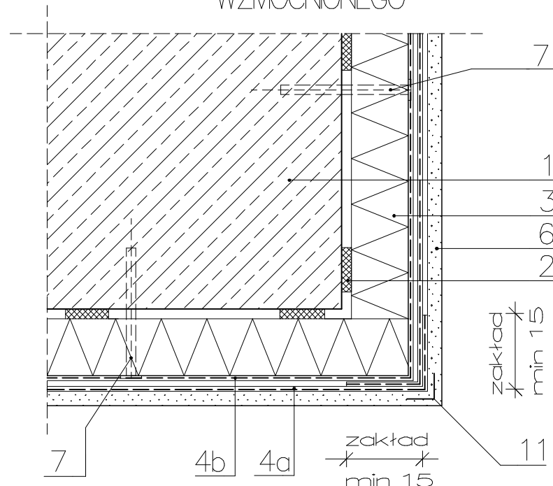
5. NAROŻE NA WYSOKOŚCI UKŁADU WZMOCNIONEGO
