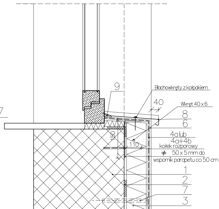
8. ZAKOŃCZENIE OCEPLENIA PRZY PARAPETACH 2 – 2
