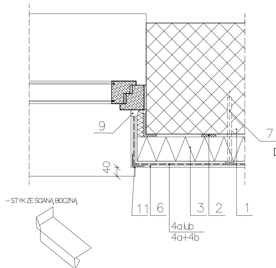
6. ZASADY PRZYKLEJANIA SIATKI ZBROJĄCEJ PRZY OTWORACH
