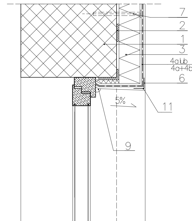
9. ZAKOŃCZENIE OCEPLENIA PRZY OŚCIEŻACH GÓRNYCH 1 – 1
