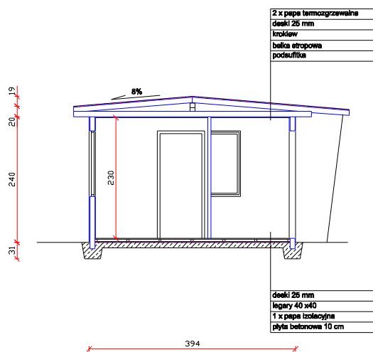
Przekrój A-A
