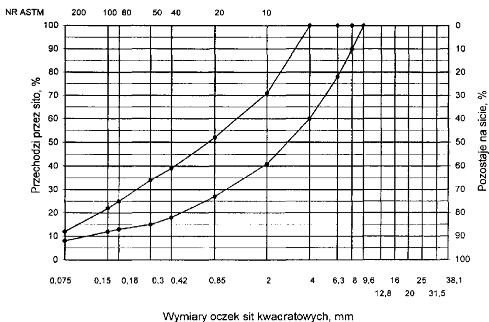
Rys. 1. Krzywe graniczne uziarnienia mieszanki mineralnej BA od 0 do 8 mm, od 0 do 6,3 mm do warstwy ścieralnej nawierzchni drogi o obciążeniu ruchem nawierzchni drogi o obciążeniu ruchem KR1 lub KR2
