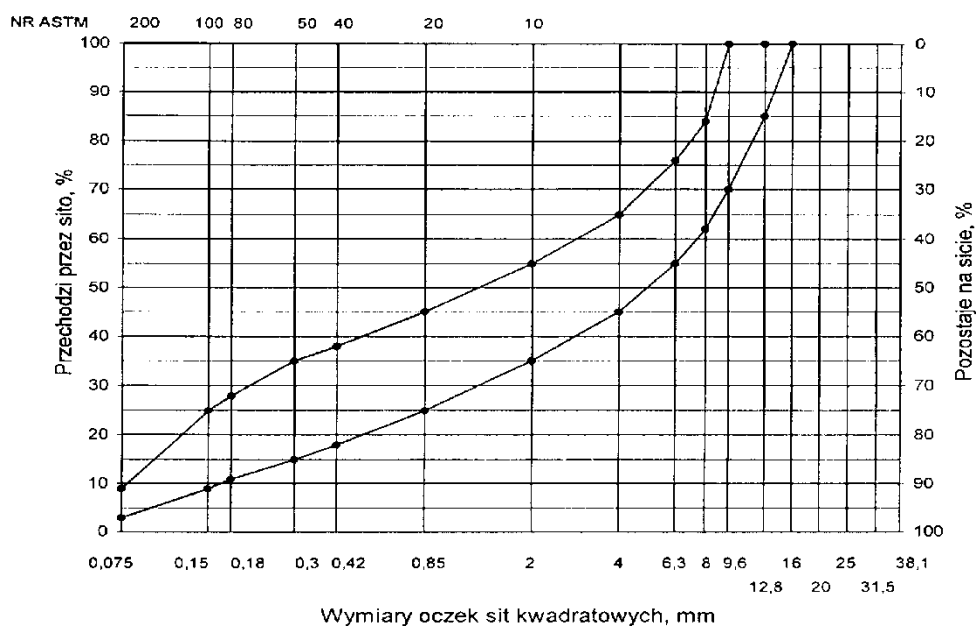
Rys. 1. Krzywe graniczne uziarnienia mieszanki mineralnej BA od 0 do 12,8 mm do warstwy wiążącej, wyrównawczej i wzmacniającej nawierzchni drogi o obciążeniu ruchem KR1 lub KR2
