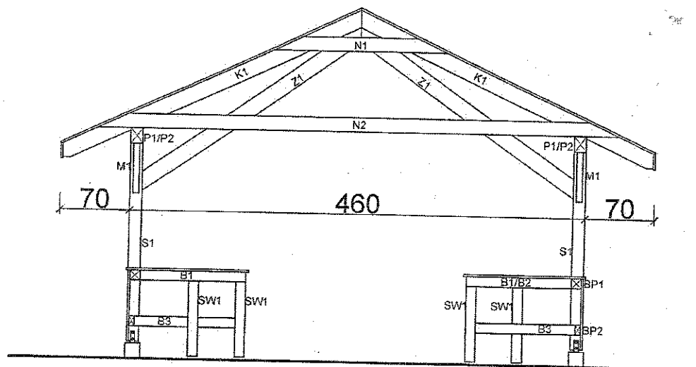
PRZEKRÓJ
