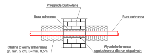
SCHEMAT PRZEJŚCIA POZ. PRZEZ PRZEGRODĘ BUDOWLANĄ RURY NIEPALNEJ
