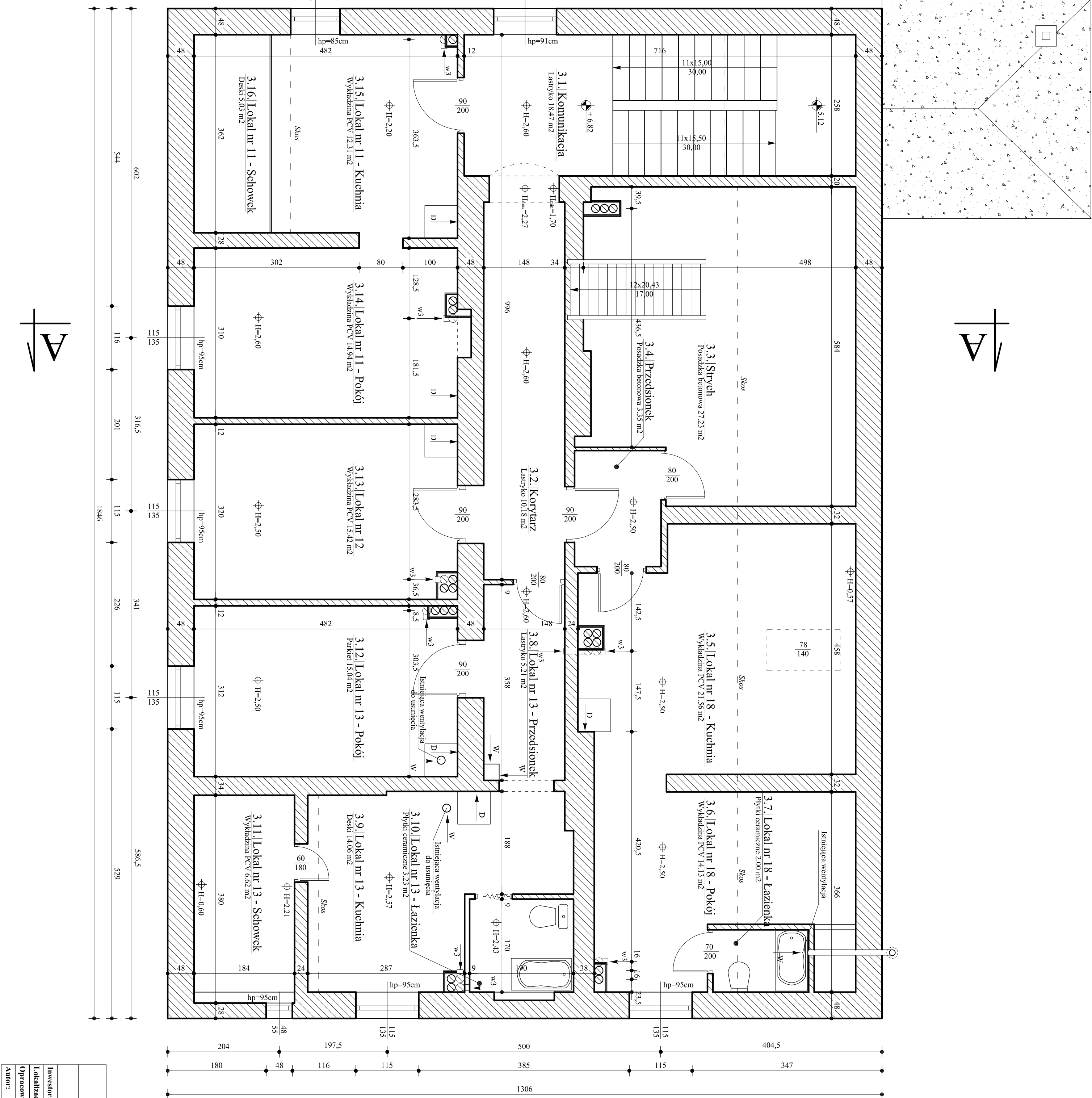
RZUT PODDASZA W5
