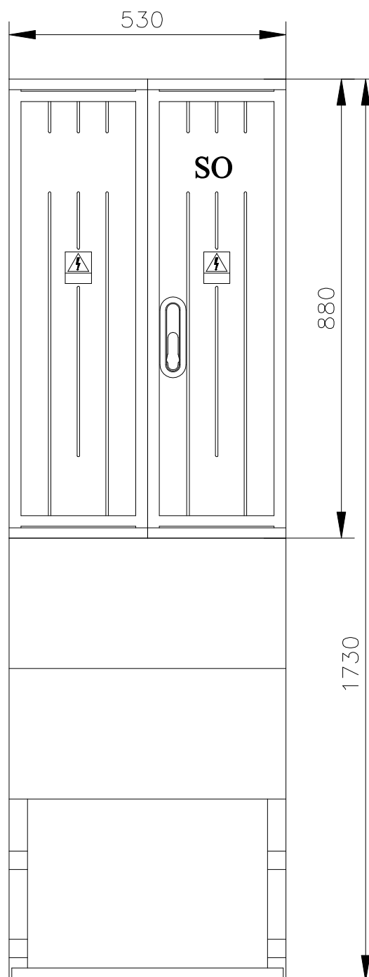
Widok elewacji szafki
