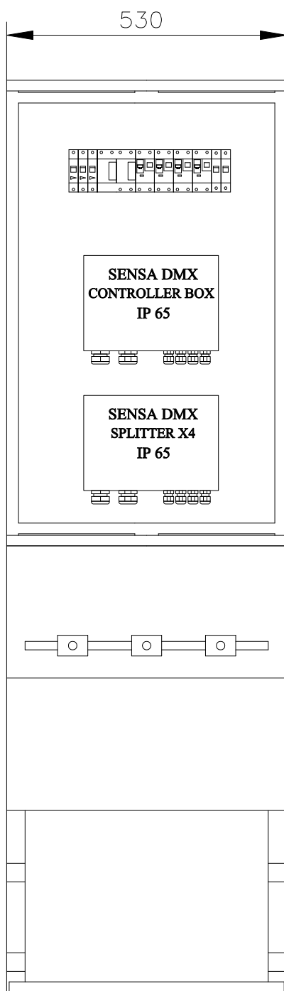
Widok elementów w szafce
