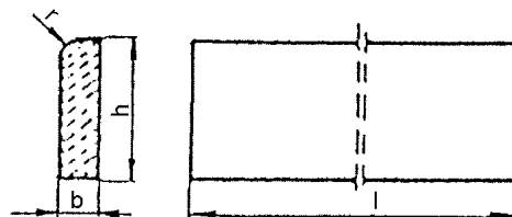
Rysunek 1. Kształt betonowego opornika betonowego
