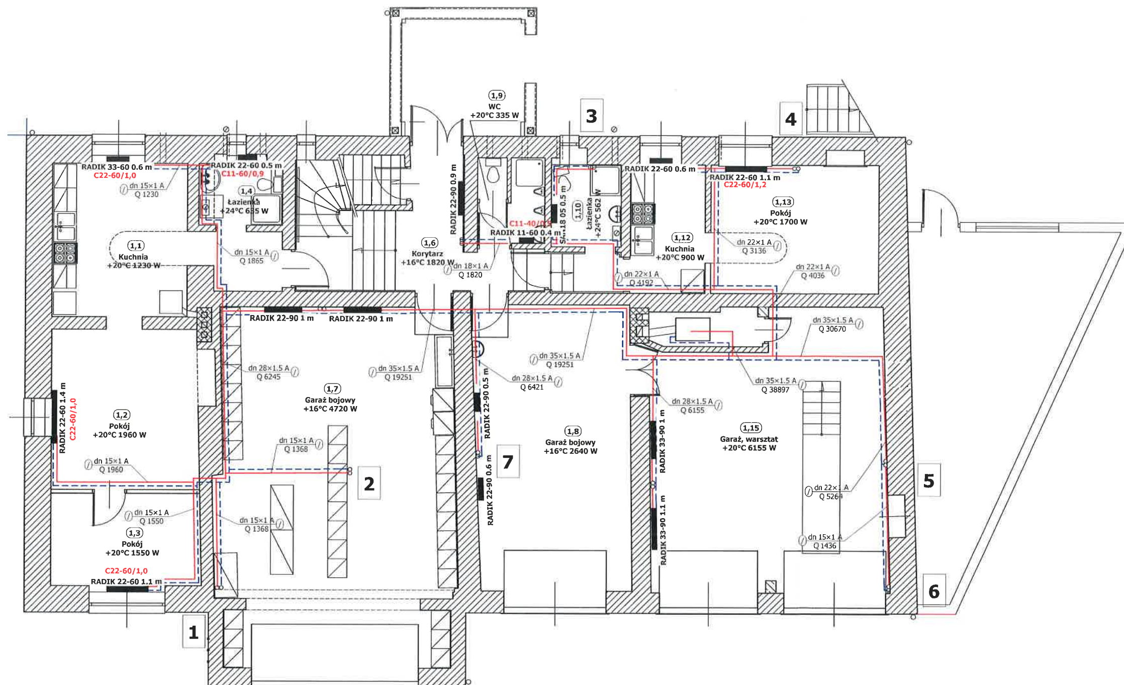
RZUT PARTERU
