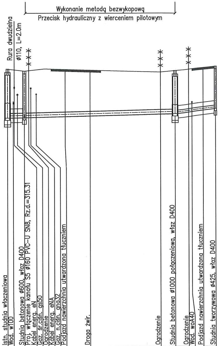
POZIOM PORÓWNAWCZY 305.00 m n.p.m.
