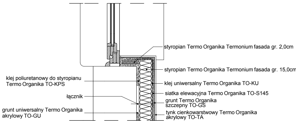
DETAL 1 Docieplenie otworu okiennego
