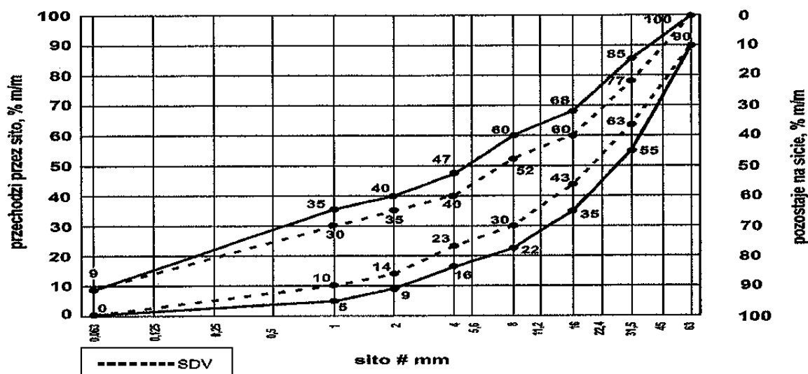
Rys. 3. Krzywe graniczne uziarnienia mieszanki kruszywa niezwiązanego 0/63 mm do warstw podbudowy zasadniczej Oprócz wymagań podanych na rysunkach od 1 do 3, wymaga się aby 90% uziarnień mieszank zbadanych w ramach ZKP w okresie 6 miesięcy spełniało wymagania kategorii podanych w tablicach 2 i 3, aby zapewnić jednorodność i ciągłość uziarnienia mieszank.
