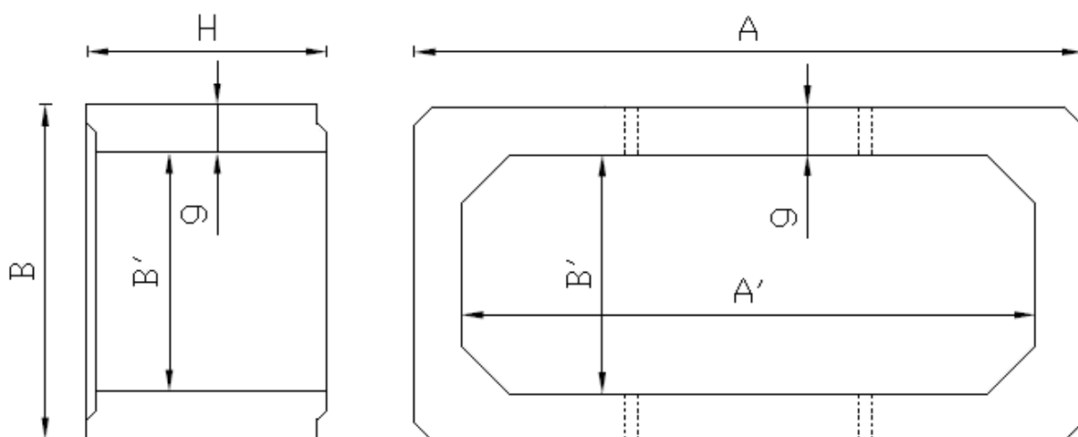
Rysunek 1. Dane techniczne przepustu. (Źródło: betonbest.pl)
